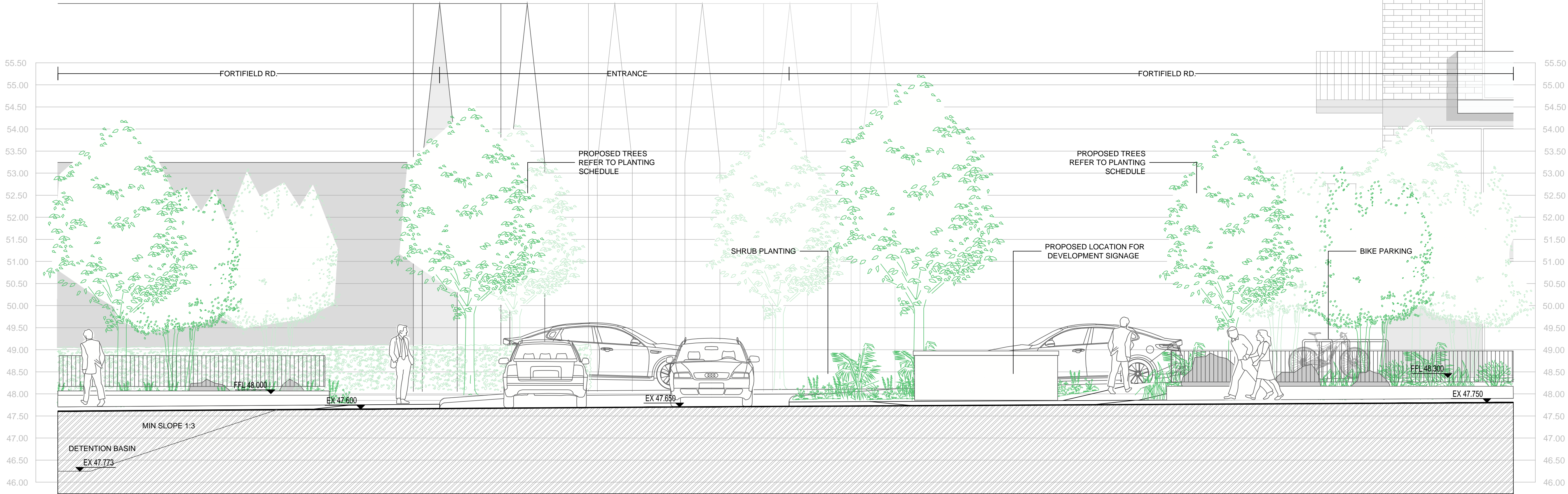
01 SECTION 1 SCALE: 1:50 @A1
