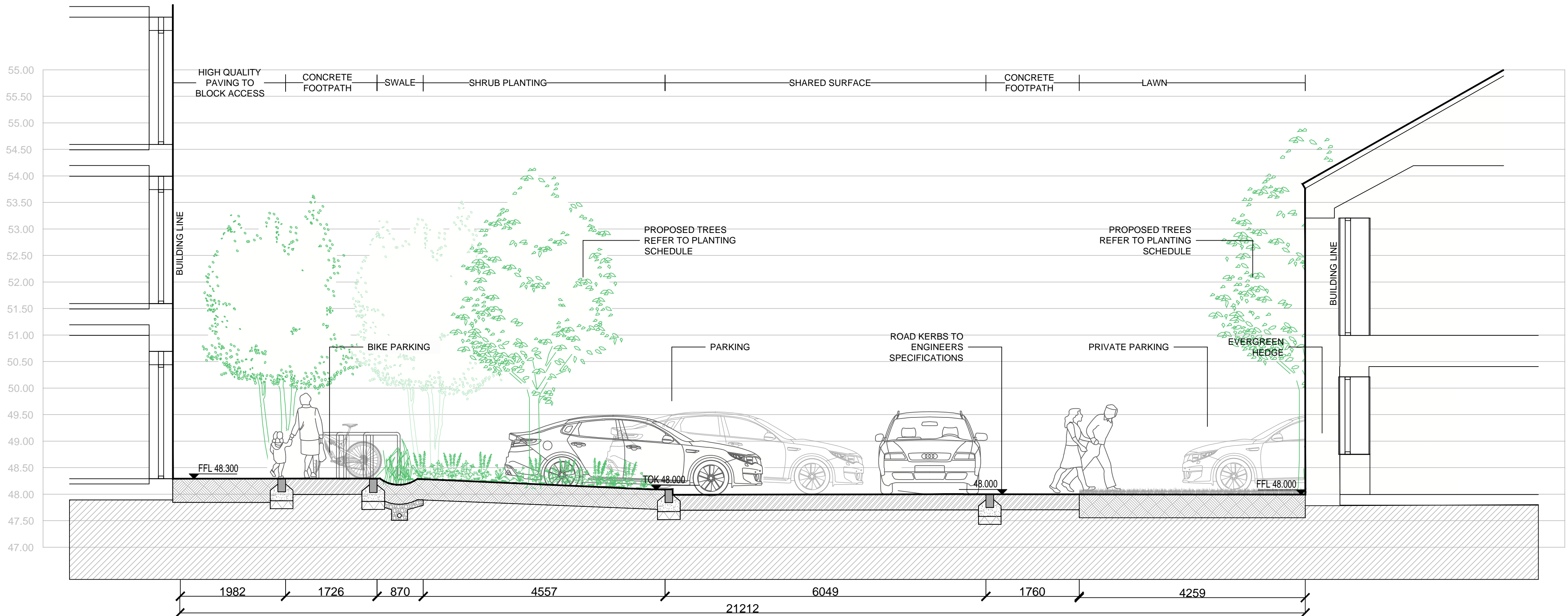
02 SECTION 2 SCALE: 1:50 @A1
