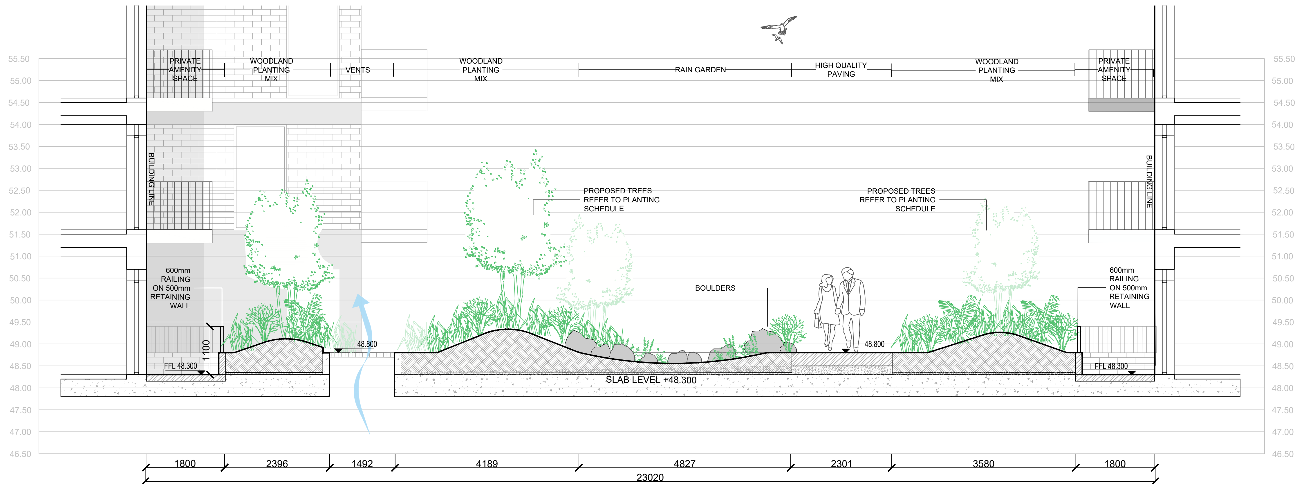
08 SECTION 8 SCALE: 1:50 @A1
