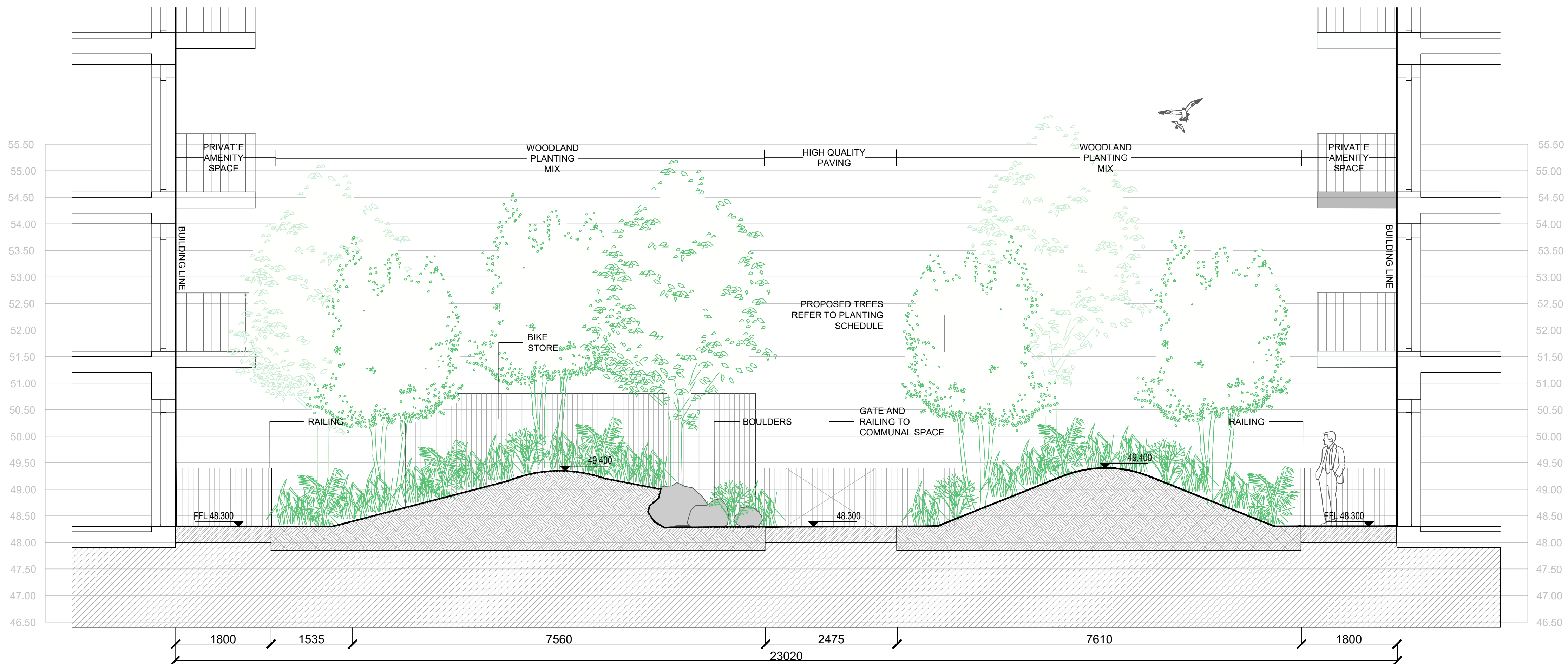
07 SECTION 7 SCALE: 1:50 @A1
