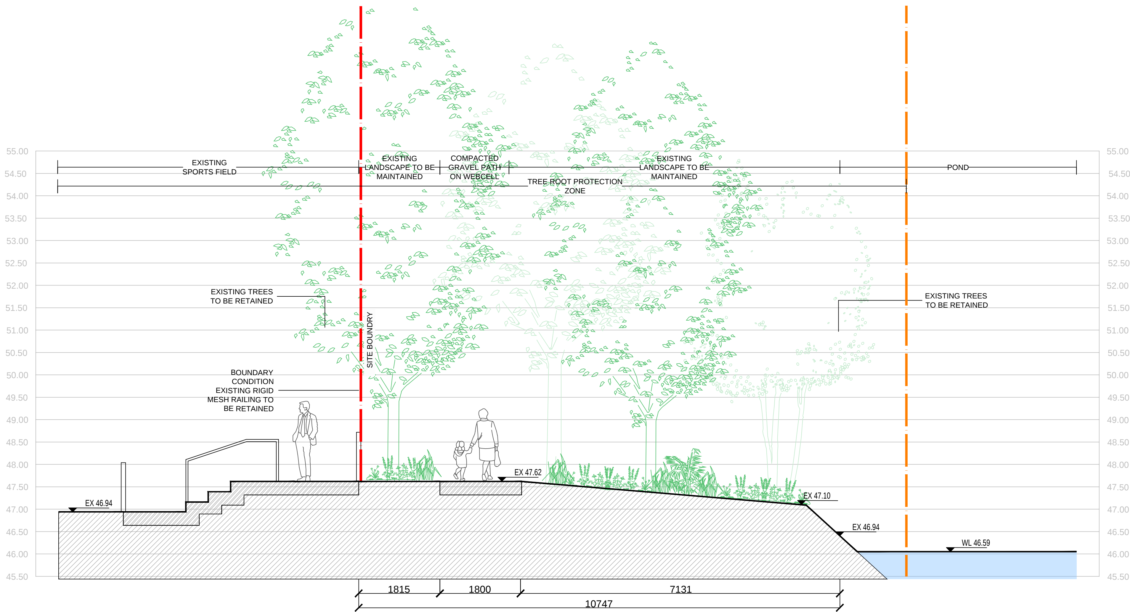
16 SECTION 16 SCALE: 1:50 @A1
