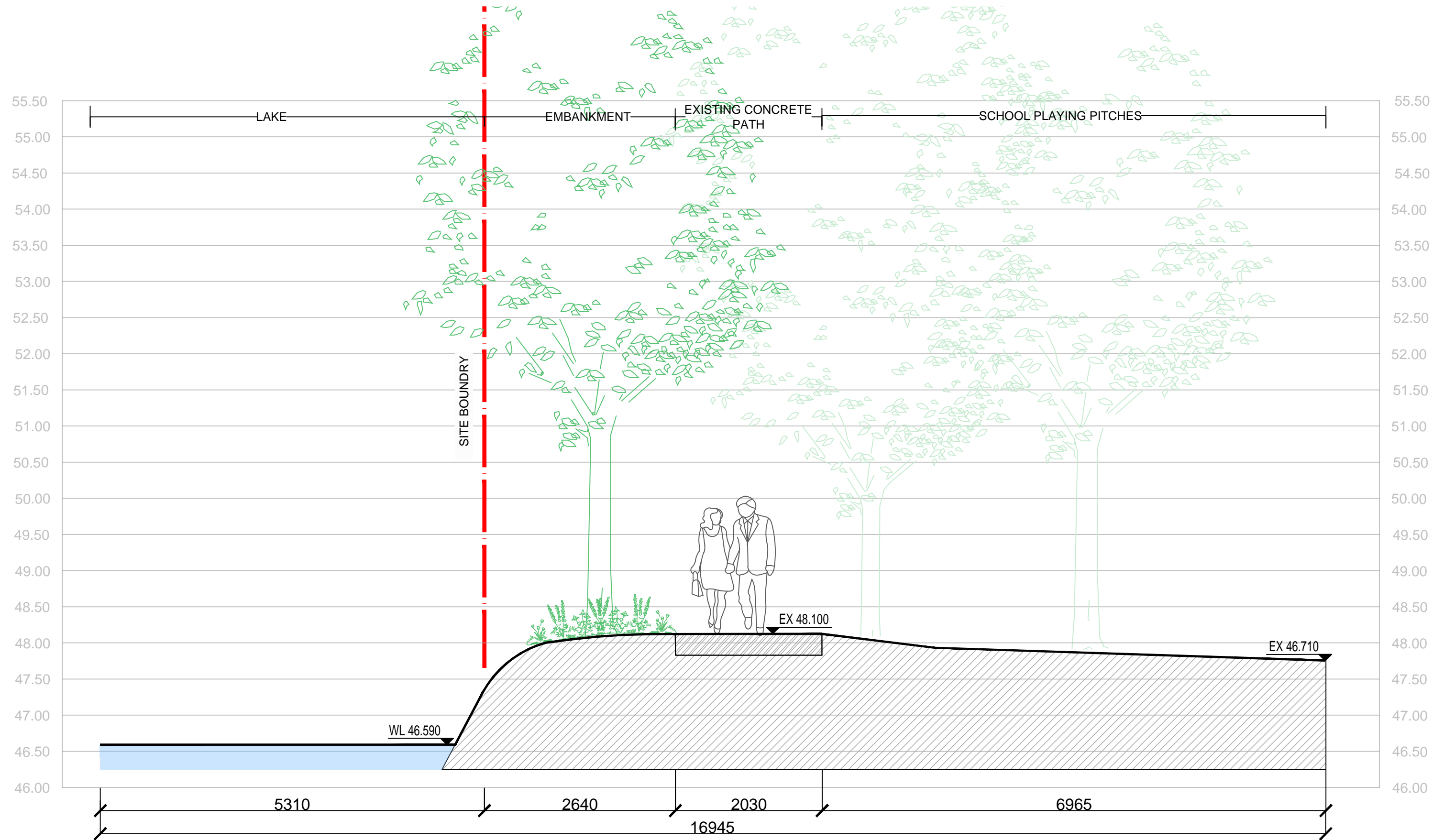
21 SECTION 21 SCALE: 1:50 @A1
